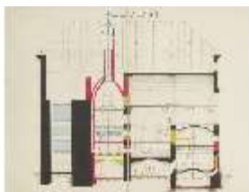
HchAS.III, Querschnitt zur Schlossbrauerei Herrenwörth, DI016510, BSV
