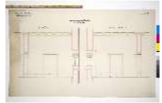
LIIMus.IV, Speisezimmer, östl. und westl. Wand, Neusch., DI031511, BSV-
