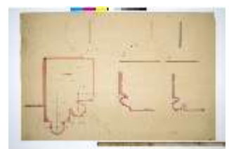
LIIMus.IV, Hauptportal, Gewände, 1. OG, Neusch., DI031312, BSV-
