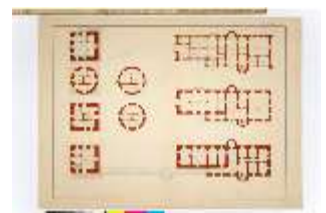
LIIMus.IV, Grundrisse, Neuschwanstein, Turm und Palas, Inv.-Nr. 1775e, DI009281, BSV-
